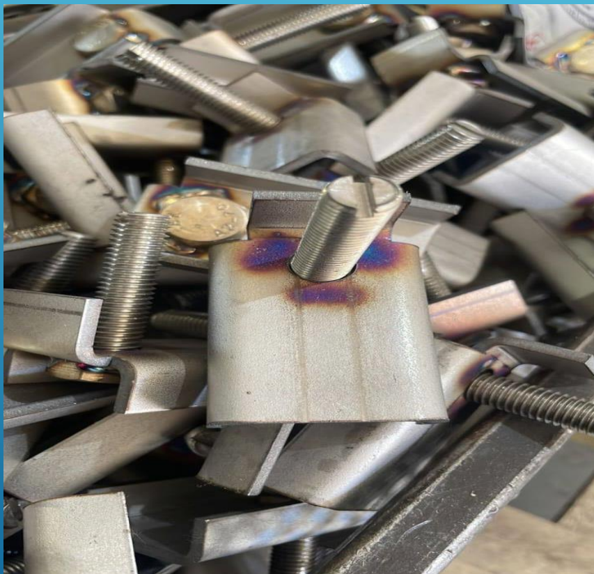
Деталь до покрытия Хим.Пас. по нержавеющей стали
